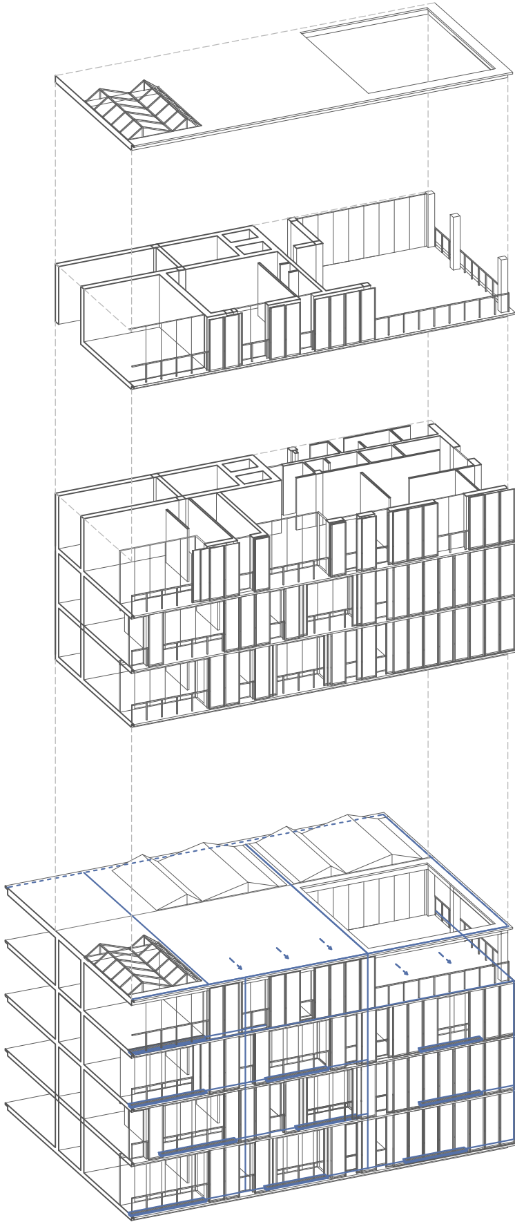
Sistema di serre interconnesse
