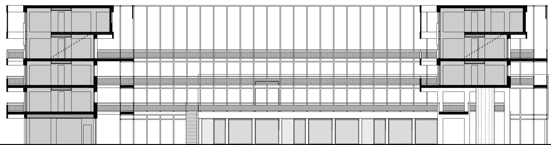
PROSPETTO - SEZIONE CC
