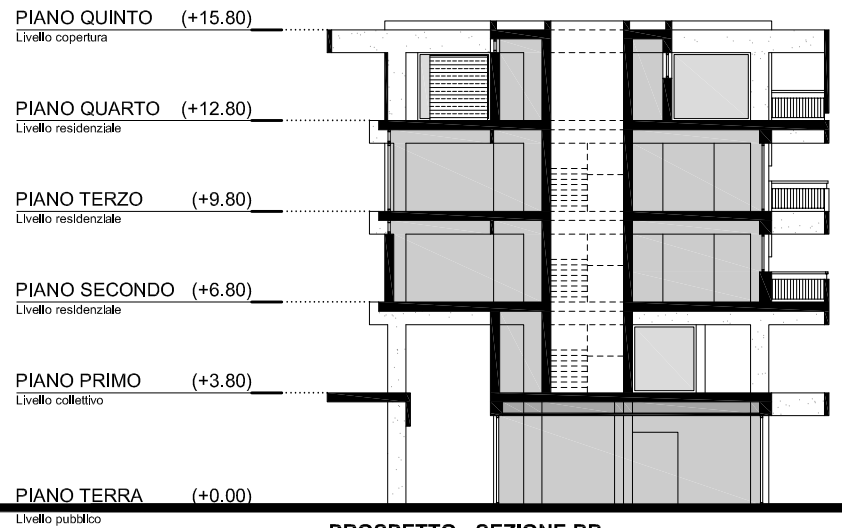
PROSPETTO - SEZIONE BB
