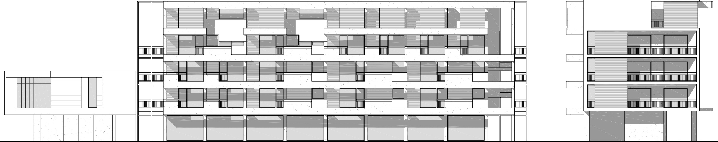
PROSPETTO - SEZIONE AA
